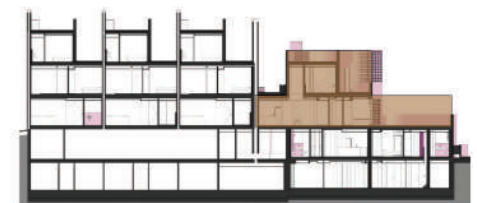
Sección Bloque 1
