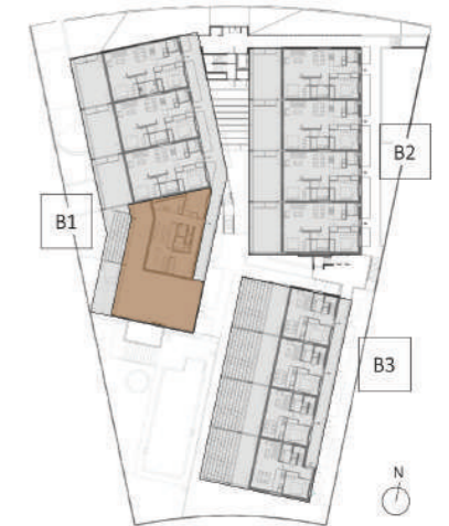
Planta Baja
